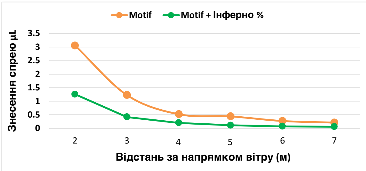
Ілюстрація 1: Silsoe Spray Applications Unit: Тест зменшення знесення: FF11003
